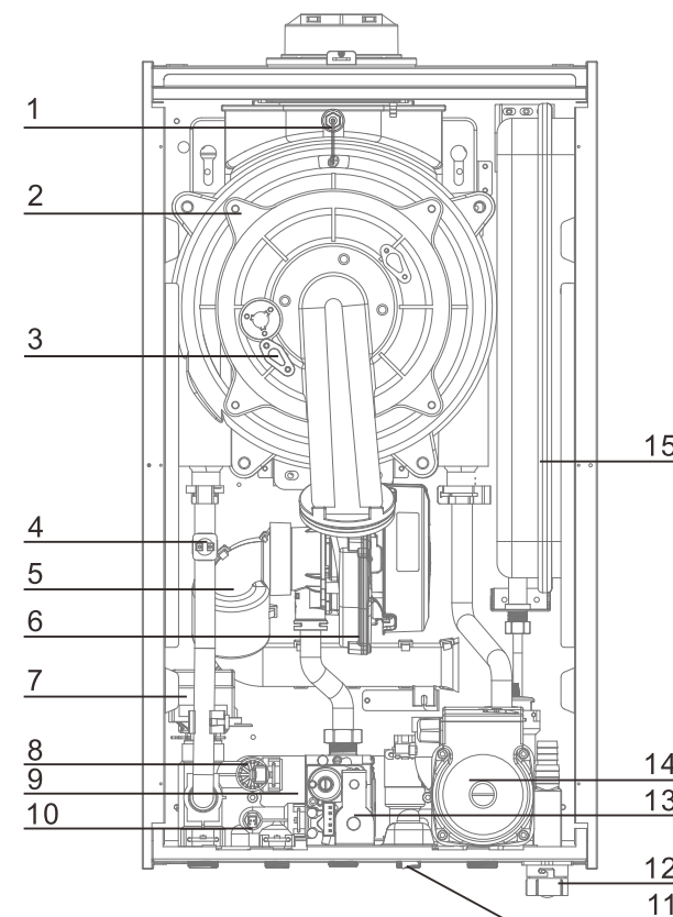
冷凝机结构示意图
