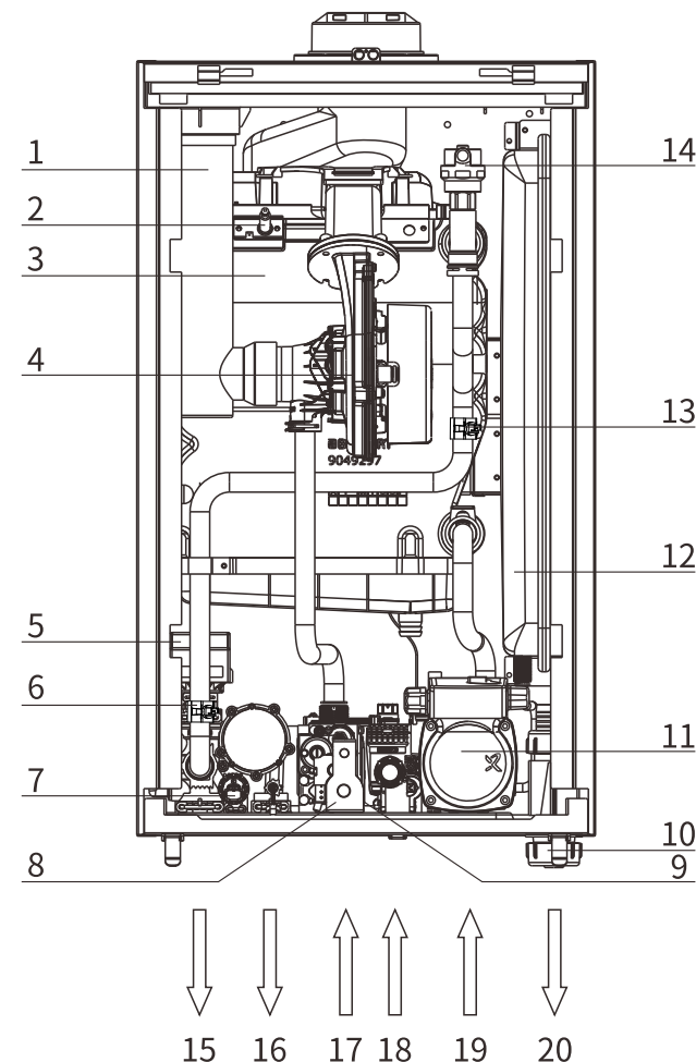
GREAT系列冷凝机结构示意图
